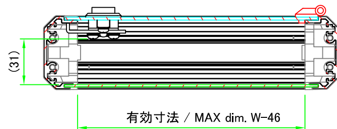
A-A ( 1 : 2.5 )
